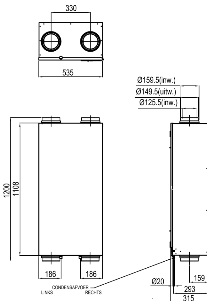
Afbeelding 0.2: Maatschets WHR 920
